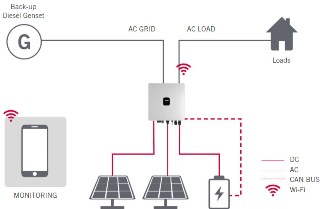
Figura 3: Instalación aislada
