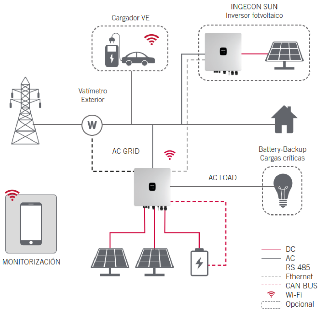
Figura 2: Instalación de autoconsumo
