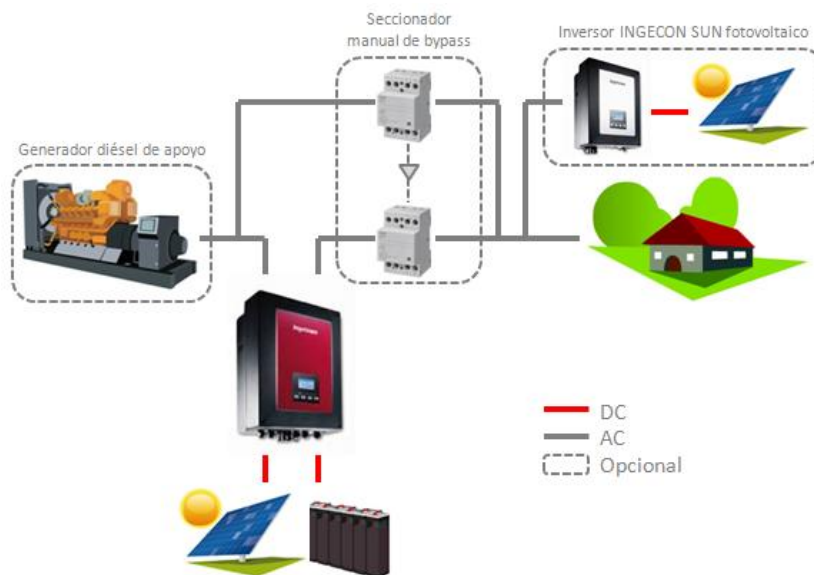
Figura 7: Instalación aislada monofásica
