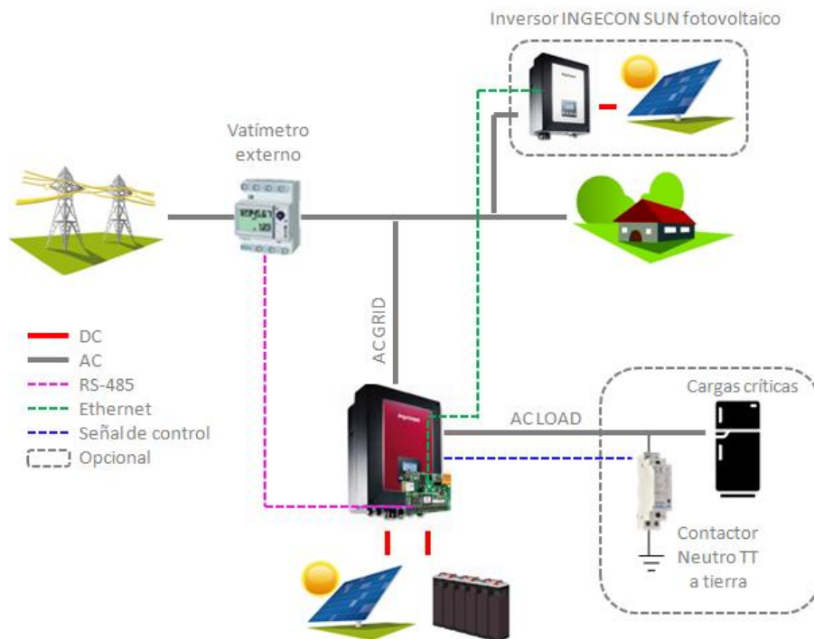
Figura 9: Instalación de autoconsumo monofásica
