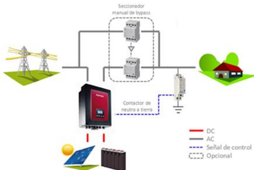
Figura 10: Instalación de autoconsumo monofásica.
